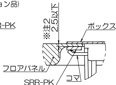
ボックス施工状態
