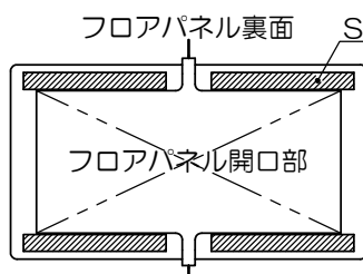
パッキン取付位置(4箇所)
