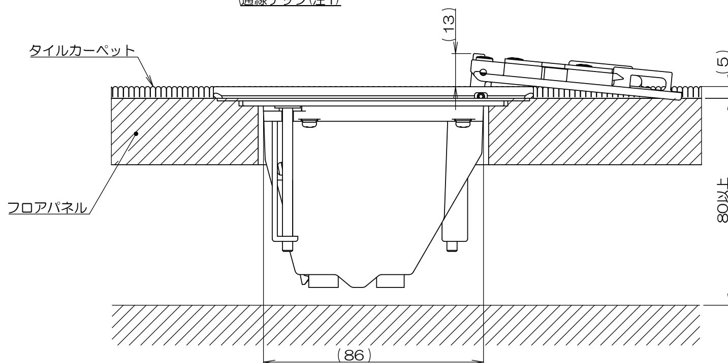
施工狀態圖
