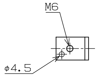
矢視A
