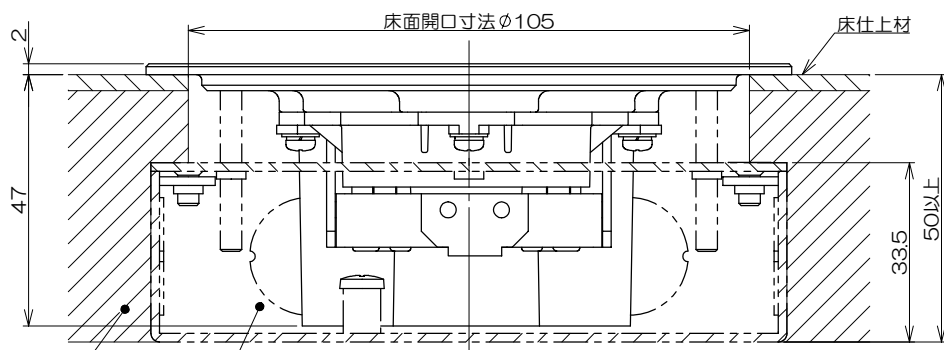
施工状態図
