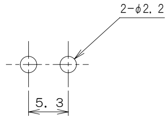
適合取付穴図
