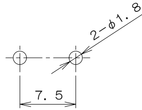
適合取付穴図
