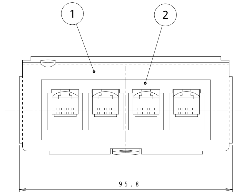
矢視 A
