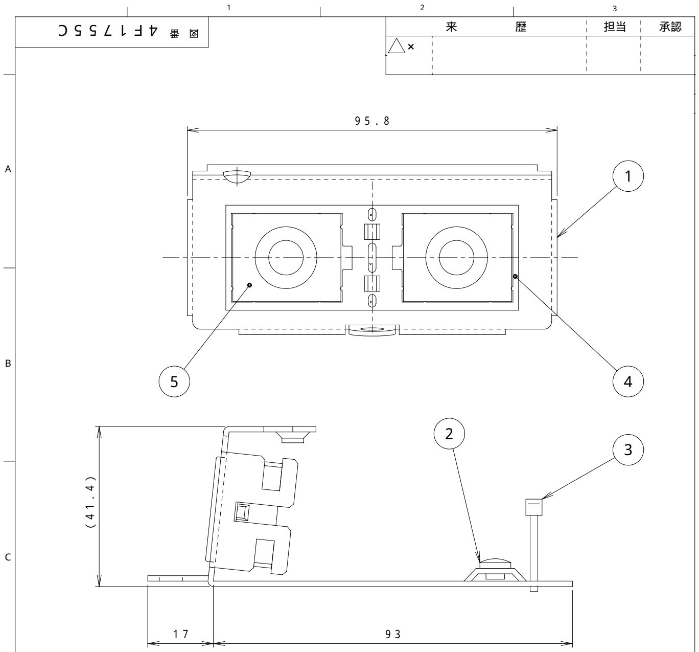
側面図
