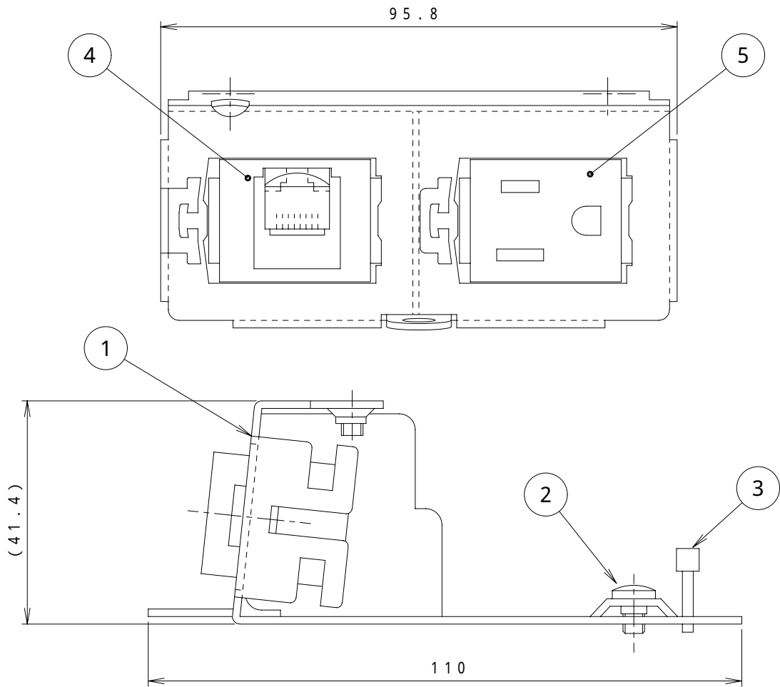
側面図
